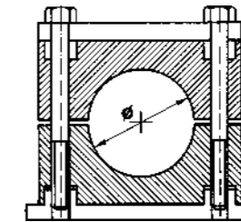
collari serie pesante heavy duty clamps
