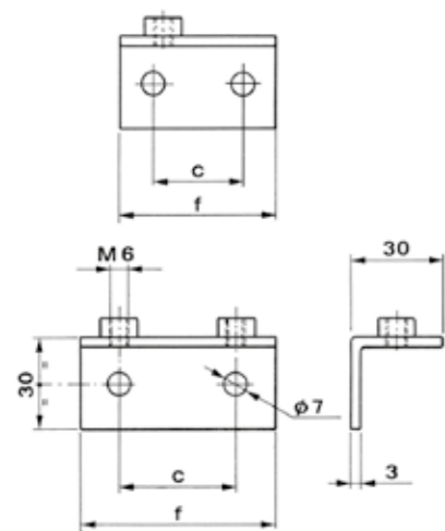
piastra ad angolo angled plate
